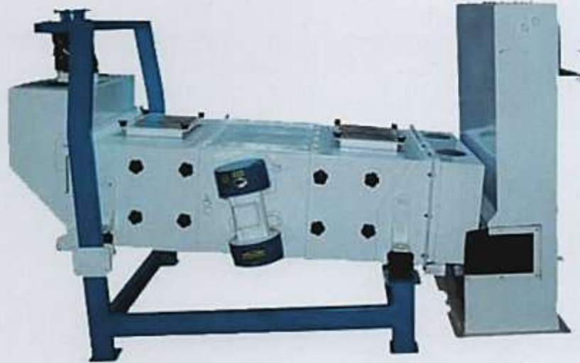
Vibro Separator
